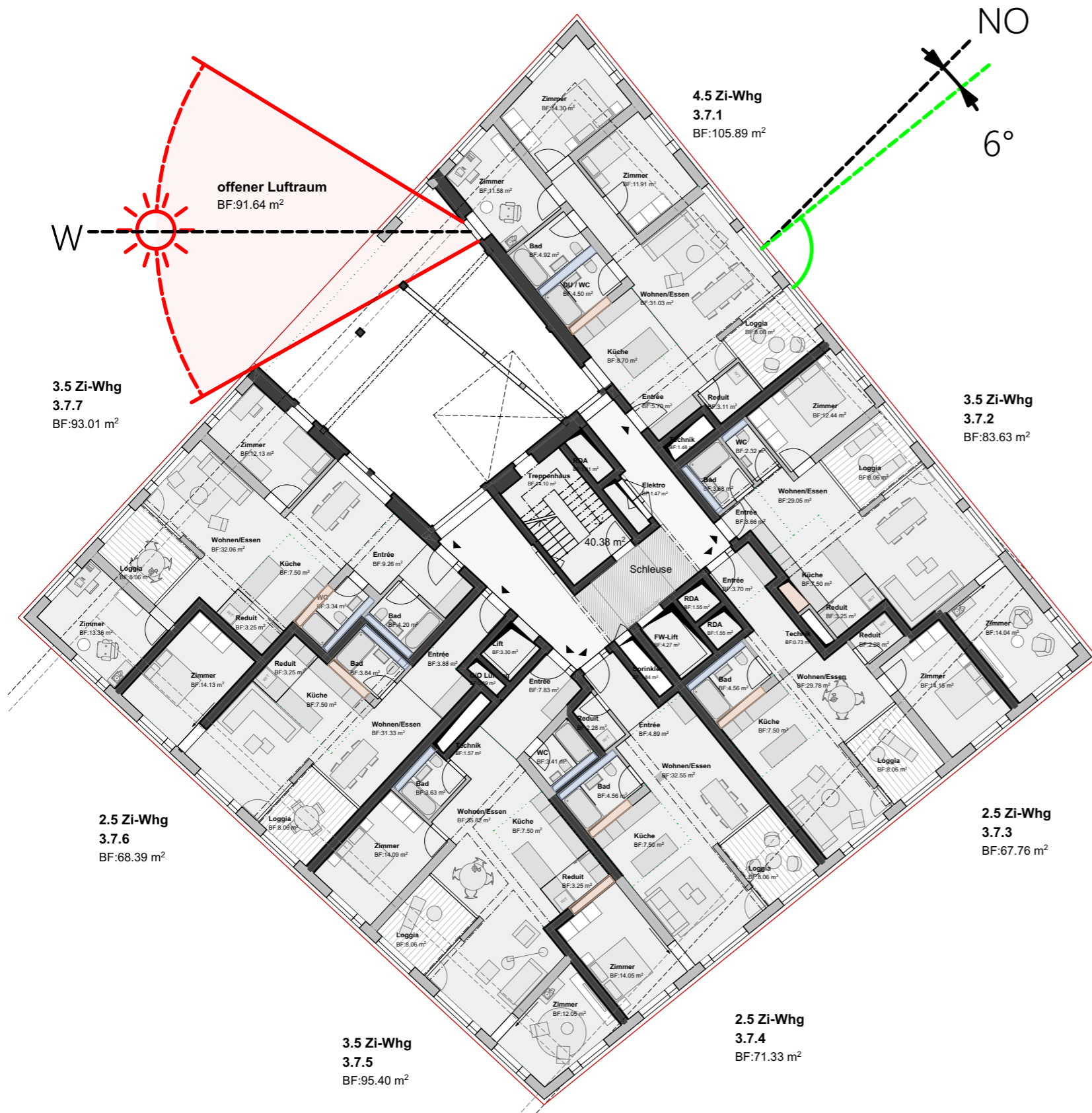
Regelgrundriss Wohnungen
