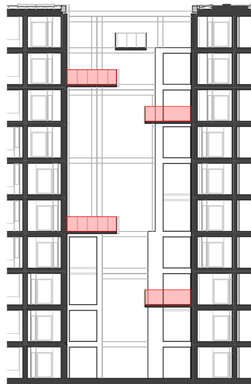
Schnitt Lüftraum B-B
