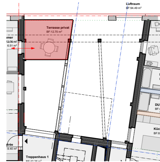
113 11. Obergeschoss
