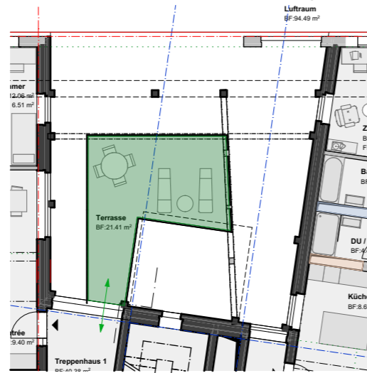
111 9. Obergeschoss
