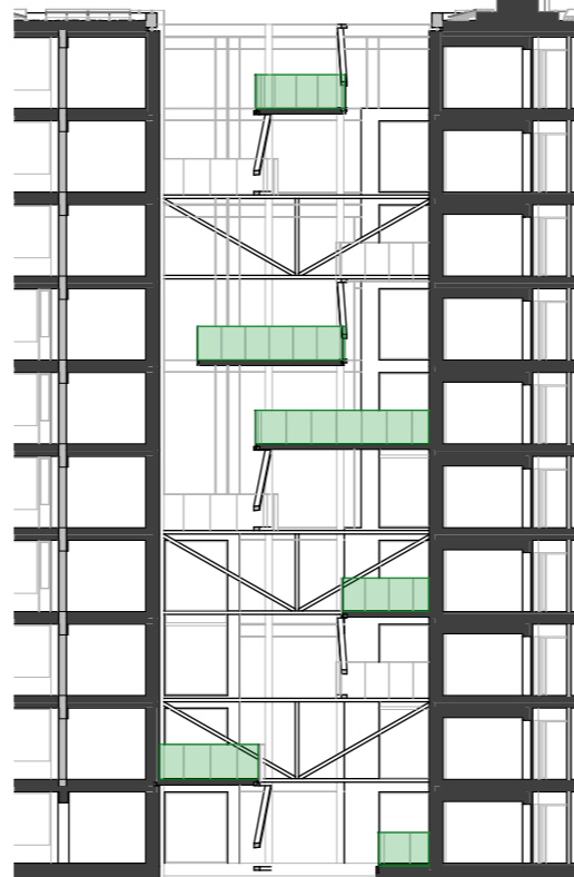
Schnitt Lüftraum C-C
