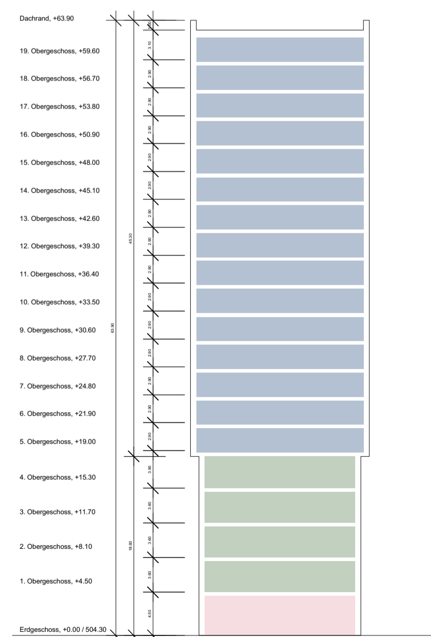
Schnitt Hochhaus (19 Obergeschosse), 1:400
