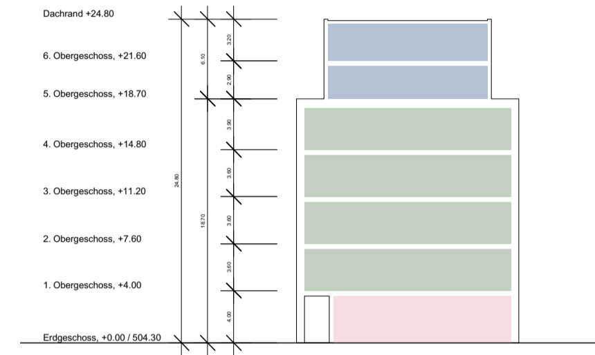
Schnitt Längsbau (6 Obergeschosse), 1:400
