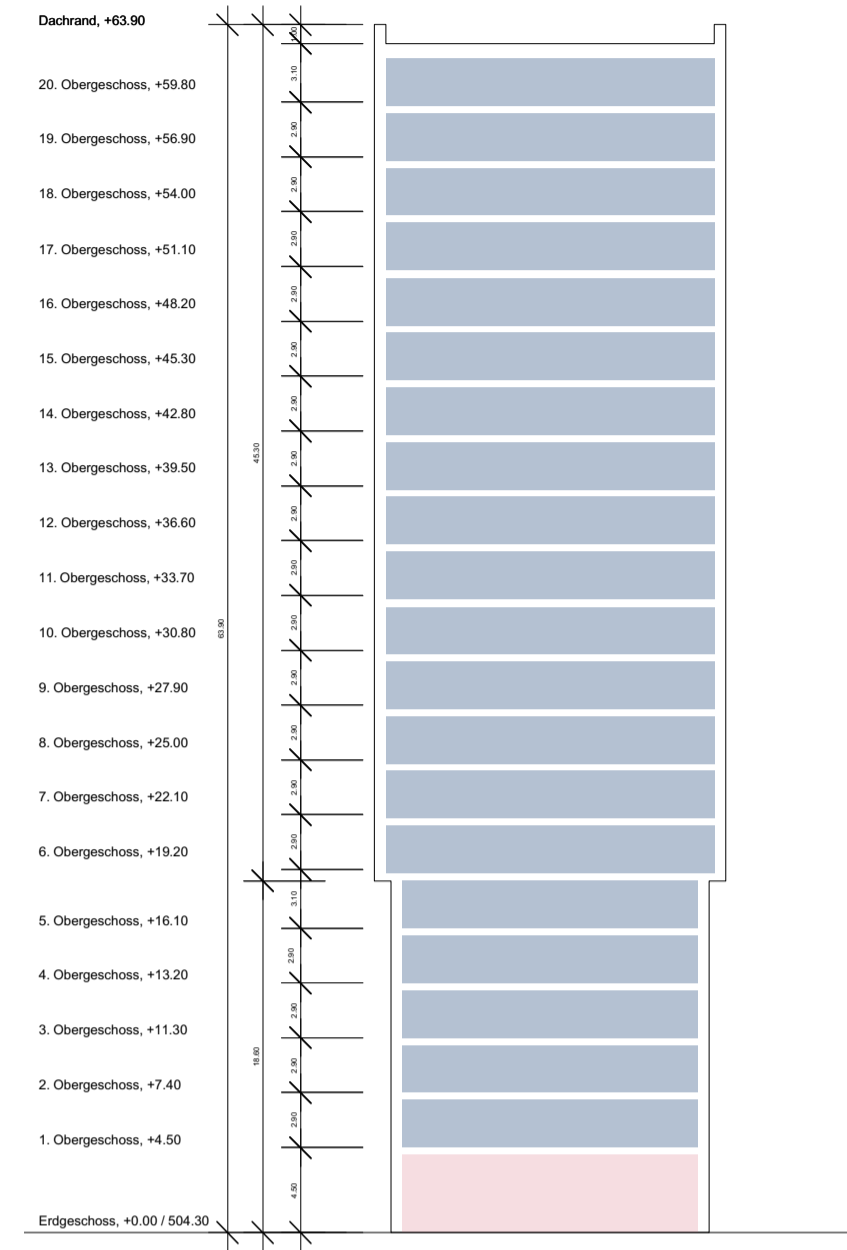
Schnitt Hochhaus (20 Obergeschosse), 1:400
