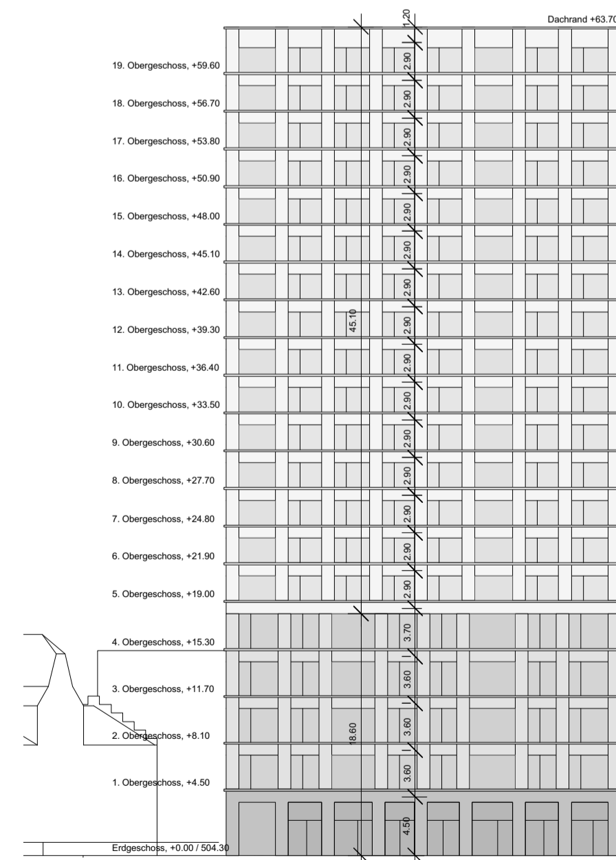
Ansicht Hochhaus + Längsbau, 1:400
