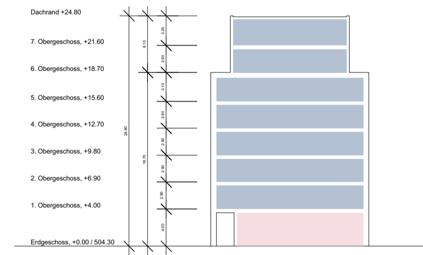
Schnitt Längsbau (7 Obergeschosse), 1:400
